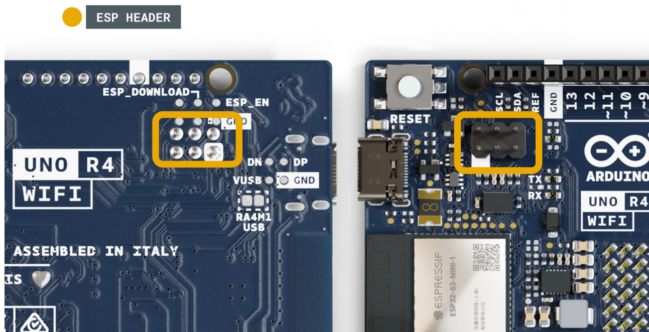
ESP引脚
